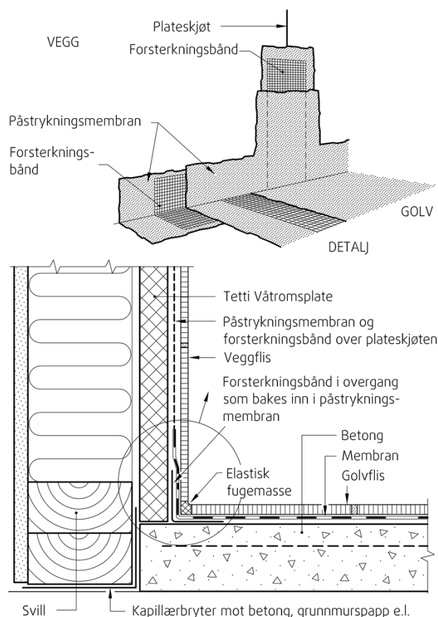
Fig. 3 Eksempel på overgang mellom flisledd golv og vegg med membran under flisene på golv.
